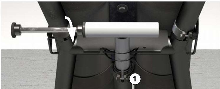
Stützbolzen einschrauben
