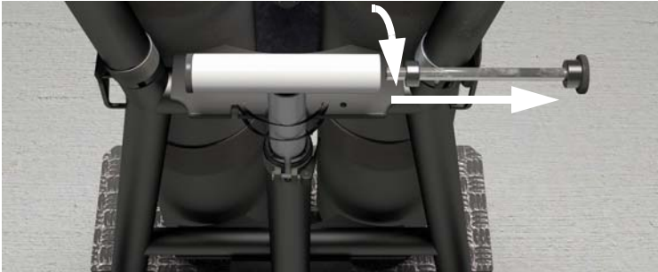
Stützbolzen herausschrauben
